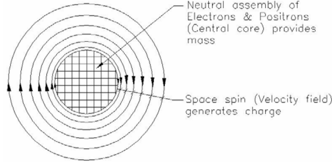
Fig. 10 Proton
